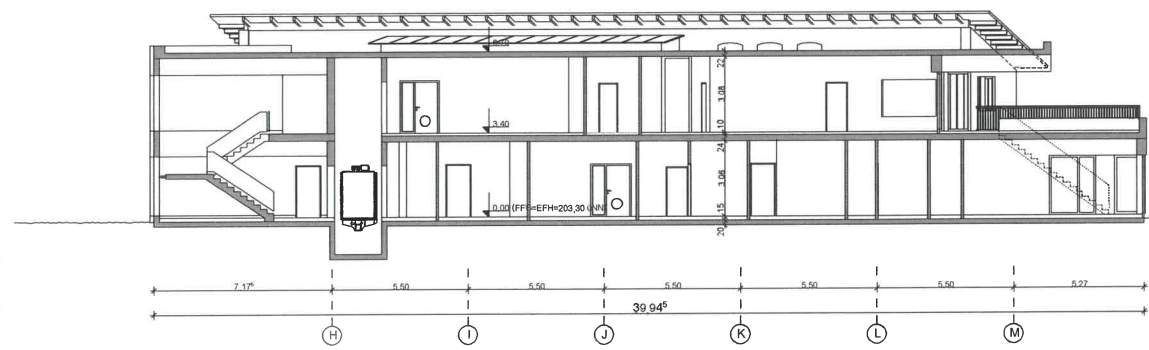
Schnitt 4-4
